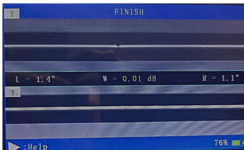
Img 3 ajuste de arco OK
